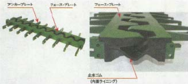
首都高羽田線に採用された「YHT-N」
