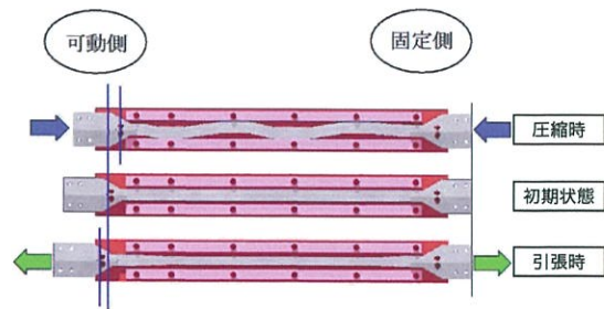
芯材降伏後の状況図
