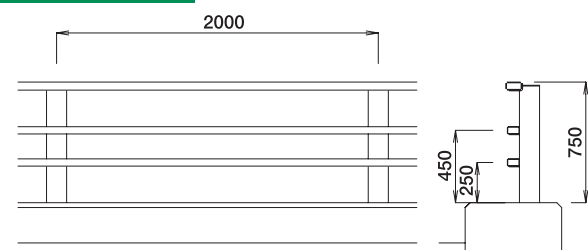
SG-Cr-3S 31.7kg/m
