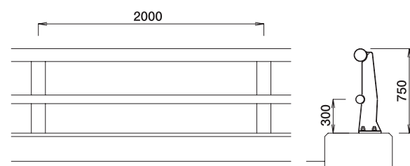
SG-Ch-2 28.9kg/m
