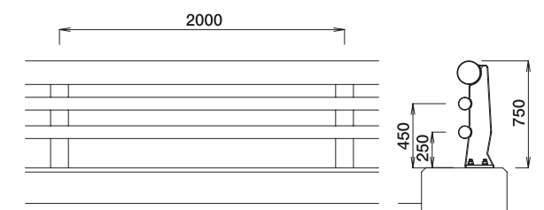
SG-Ah-3 48.2kg/m
