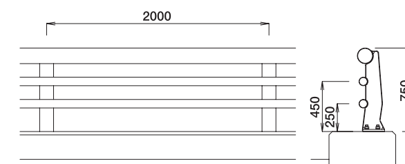
SG-Bh-3 36.4kg/m
